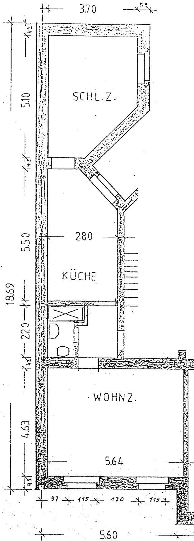
1+2 OBERGESCHOSS
